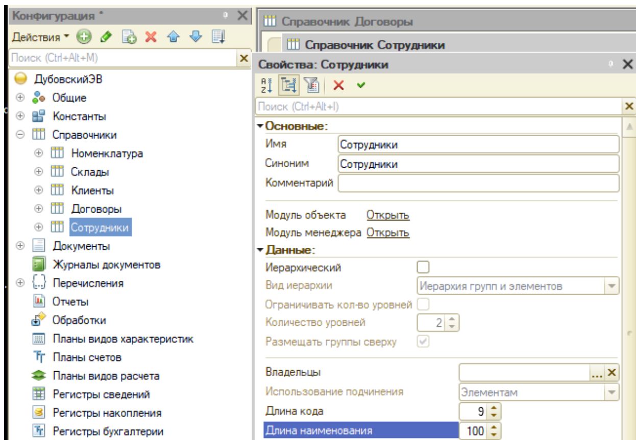
Рисунок 19 – Создание и настройка справочника “Сотрудники”
