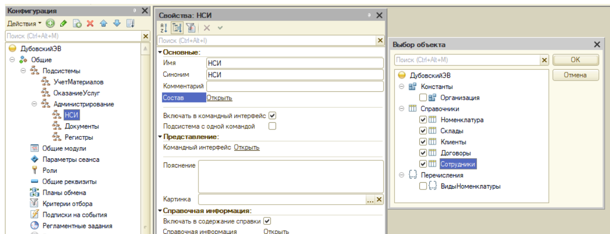
Рисунок 25 – Включение всех справочников в состав подсистемы “НСИ”
