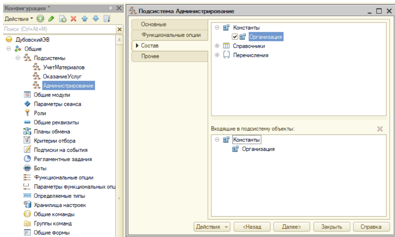
Рисунок 23 – Создание и настройка подсистемы “Администрирование”
