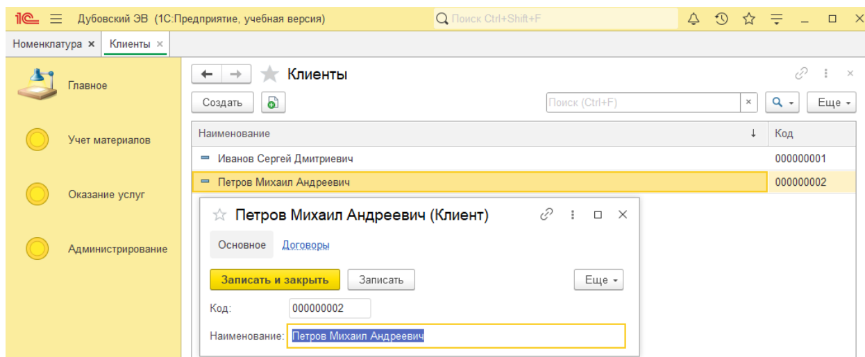
Рисунок 30 – Создание клиентов
