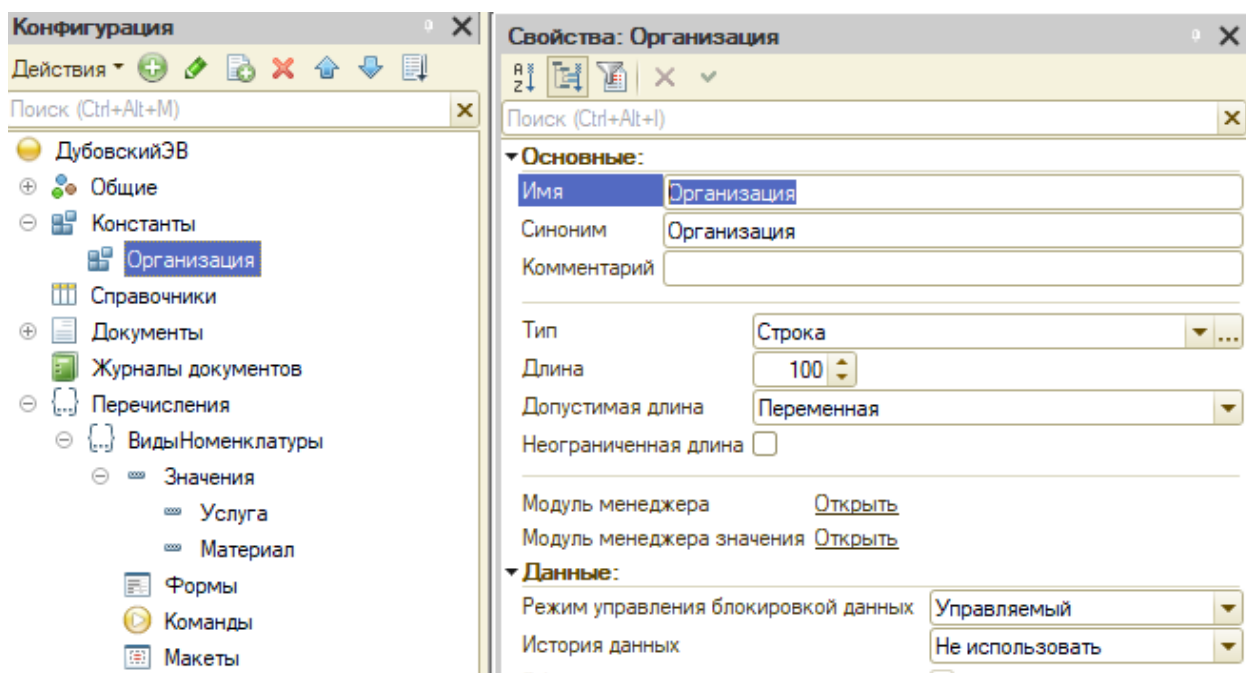
Рисунок 6 – Создание константы и перечислений
