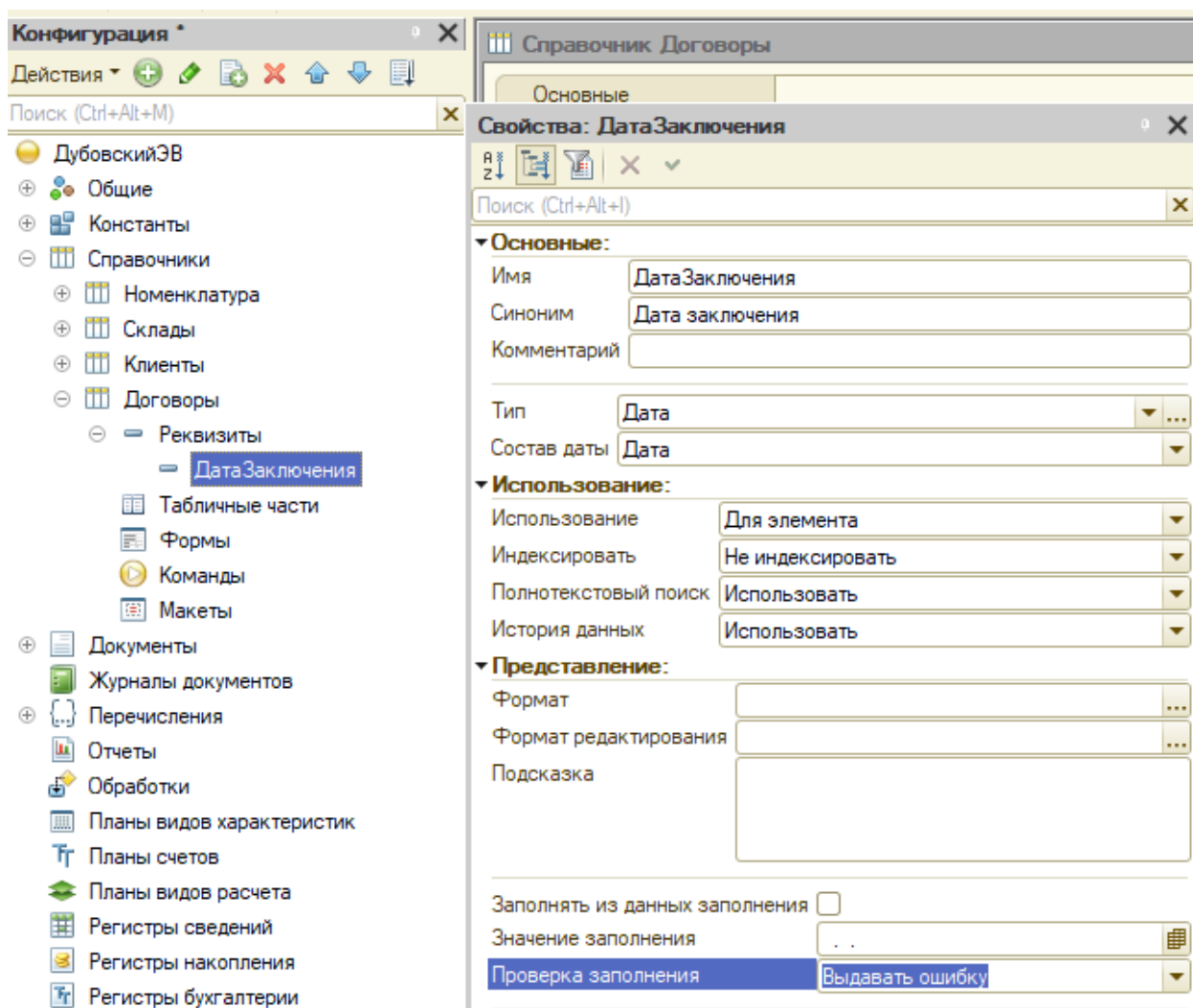
Рисунок 18 – Создание и настройка реквизита справочника “Договоры”
