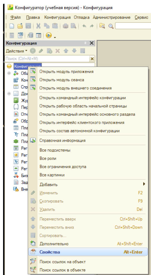
Рисунок 4 – Свойства конфигуратора
